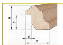
Glas- und Füllungsleisten massiv, Ramin / Eiche / Kiefer / Fichte / Buche / Mahagoni
