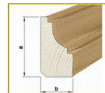
Sockelleisten, Kiefer / Fichte
